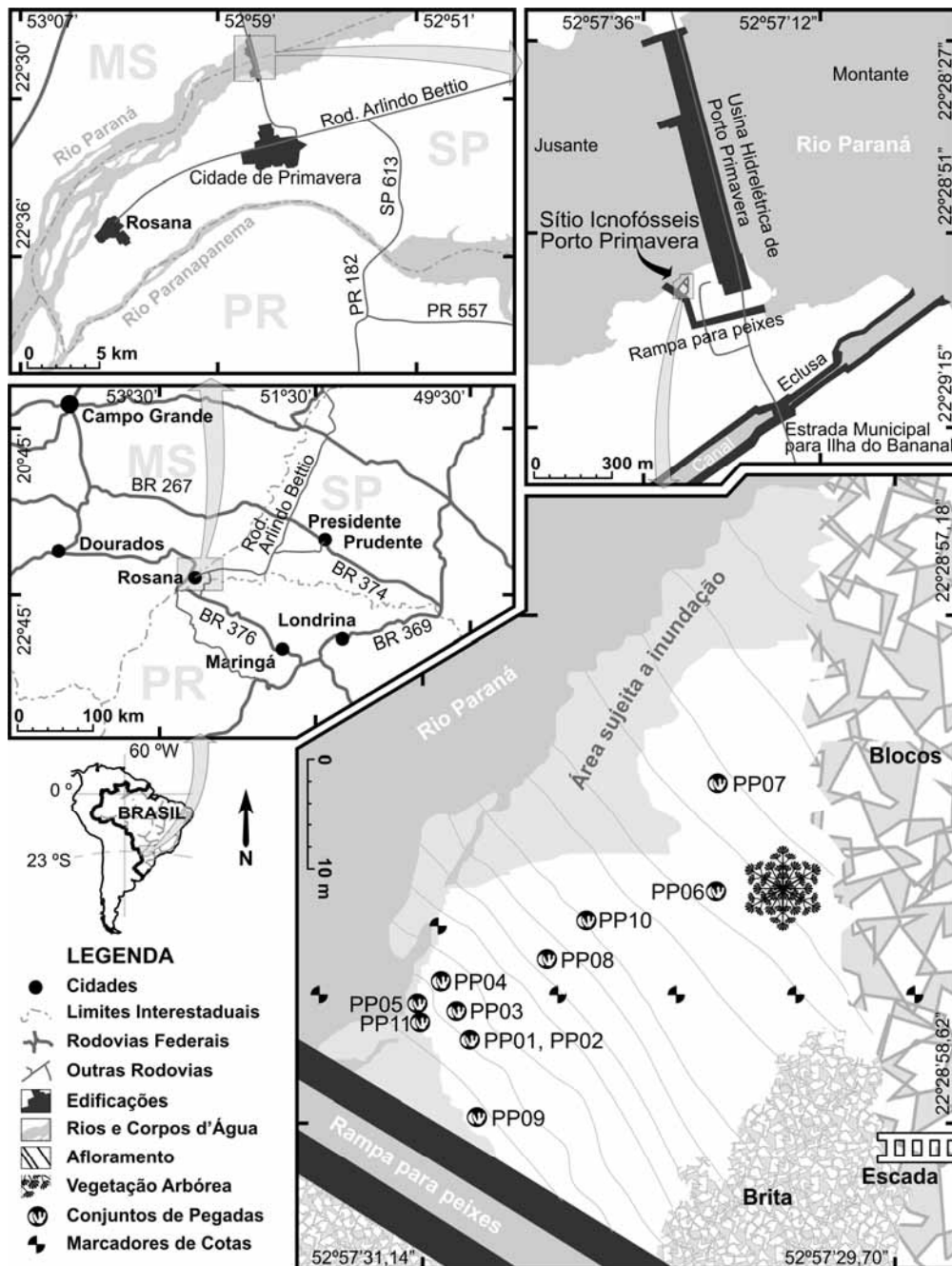
Figura 2: Mapas de localização regional e de detalhe, com posição dos icnofósseis de Porto Primavera. Figure 2: Regional and detail location maps, with the position of Porto Primavera ichnofossils.
