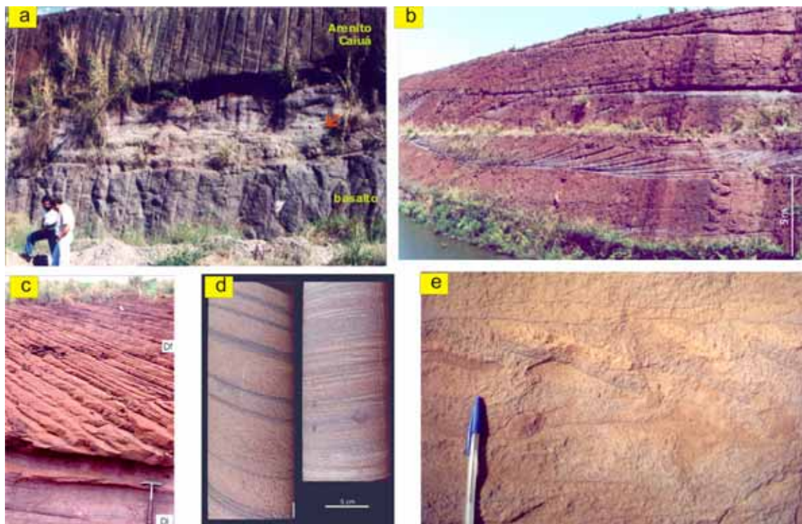
Figura 6: a) contato inferior da Formação Rio Paraná/Grupo Caiuá com basalto. Na base da unidade, abaixo dos arenitos com estratificação cruzada ocorre brecha arenosa imatura, maciça, com clastos angulosos de basalto, nódulos de argila e cimento carbonático. Ombreira esquerda da UHE Porto Primavera, próximo da ocorrência dos icnofósseis (foto da época da construção da barragem); b) Vista geral de arenitos com estratificação cruzada de grande porte, de depósitos frontais de dunas, da parte central do deserto Caiuá , Formação Rio Paraná; c) Detalhe da Formação Rio Paraná, com depósitos de partes frontais de grandes dunas (litofácies Df) e de interdunas (Di), UHE Porto Primavera, SP; d) Formação Rio Paraná, laminação característica de arenitos eólicos (testemunhos de sondagens da construção da UHE Porto Primavera); e) fragmentos rotacionados de brechas intraformacionais de gravidade (deslizamentos de partes frontais de dunas), indicativos de umidade no ambiente desértico, Formação Rio Paraná.
