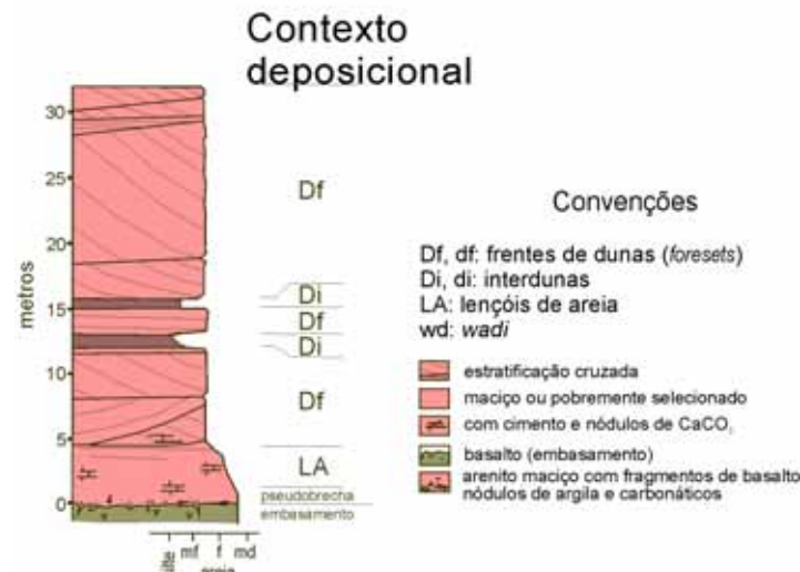
Figura 5: Seção-tipo da Formação Rio Paraná, U.H.E. Porto Primavera, Pontal do Paranapanema (São Paulo). Figure 5: Rio Paraná Formation type-section, Porto Primavera Hydroelectric Plant, Pontal do Paranapanema (São Paulo State
