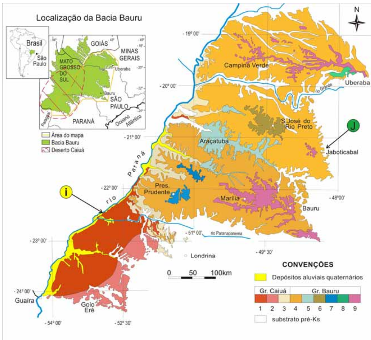
Figura 3. Mapa geológico da parte oriental da Bacia Bauru. Figure 3. Geological map of the Bauru Basin eastern part.
