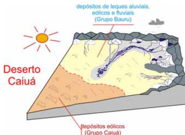
Figura 4. Contexto deposicional da parte oriental da Bacia Bauru. Figure 4. Depositional setting of the Bauru Basin eastern part.
