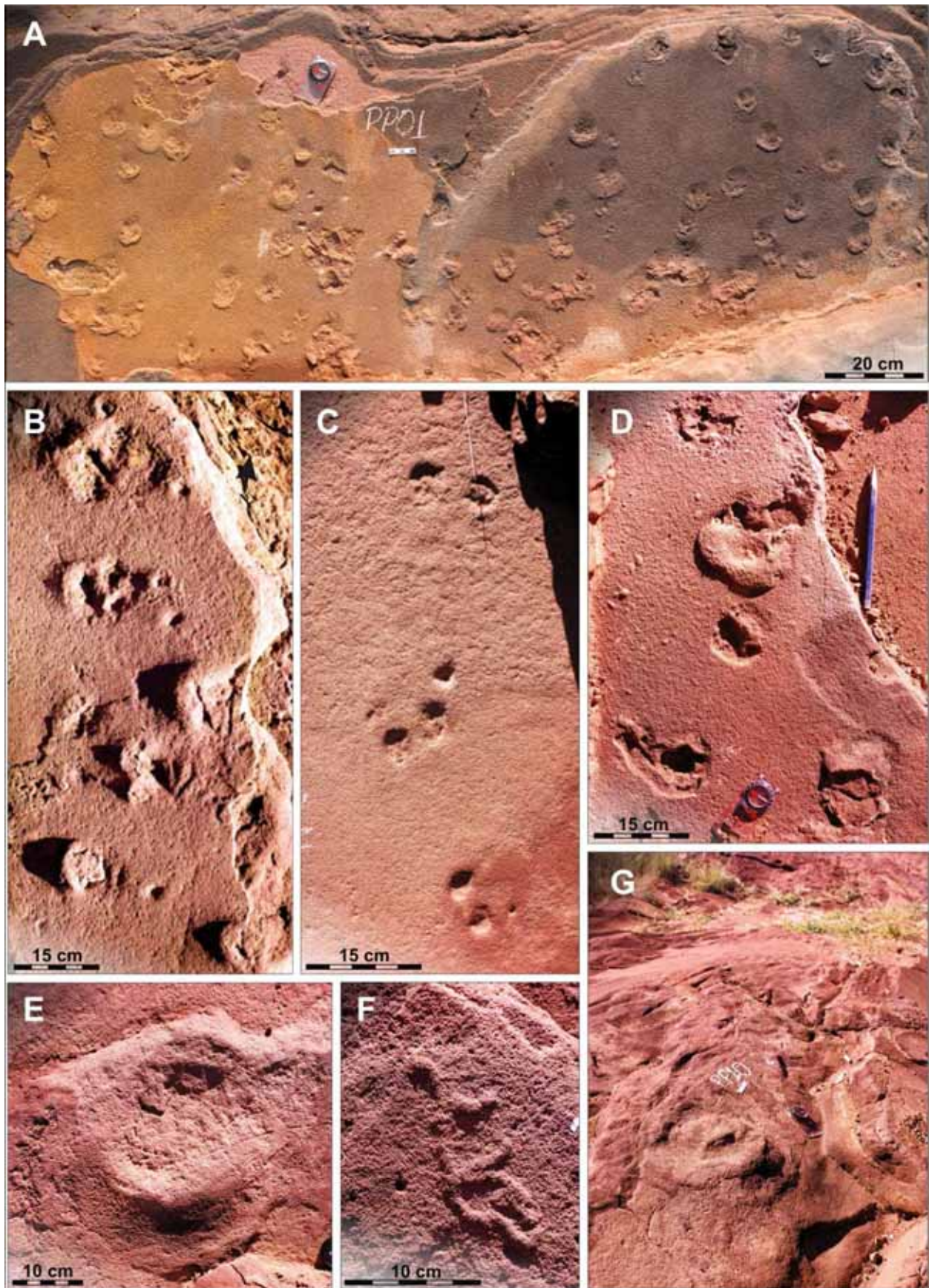
Figura 7: Icnofósseis em depósitos frontais de dunas, arenitos da Formação Rio Paraná. UHE Porto Primavera, SP. Figure 7: Ichnofossils on forests dune deposits, Rio Paraná Formation sandstones, Paraná River. Porto Primavera Hydroelectric Plant, Brazil.
