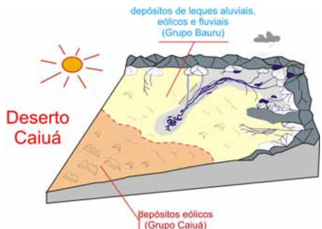
Figura 4. Contexto deposicional da parte oriental da Bacia Bauru. Figure 4. Depositional setting of the Bauru Basin eastern part.
