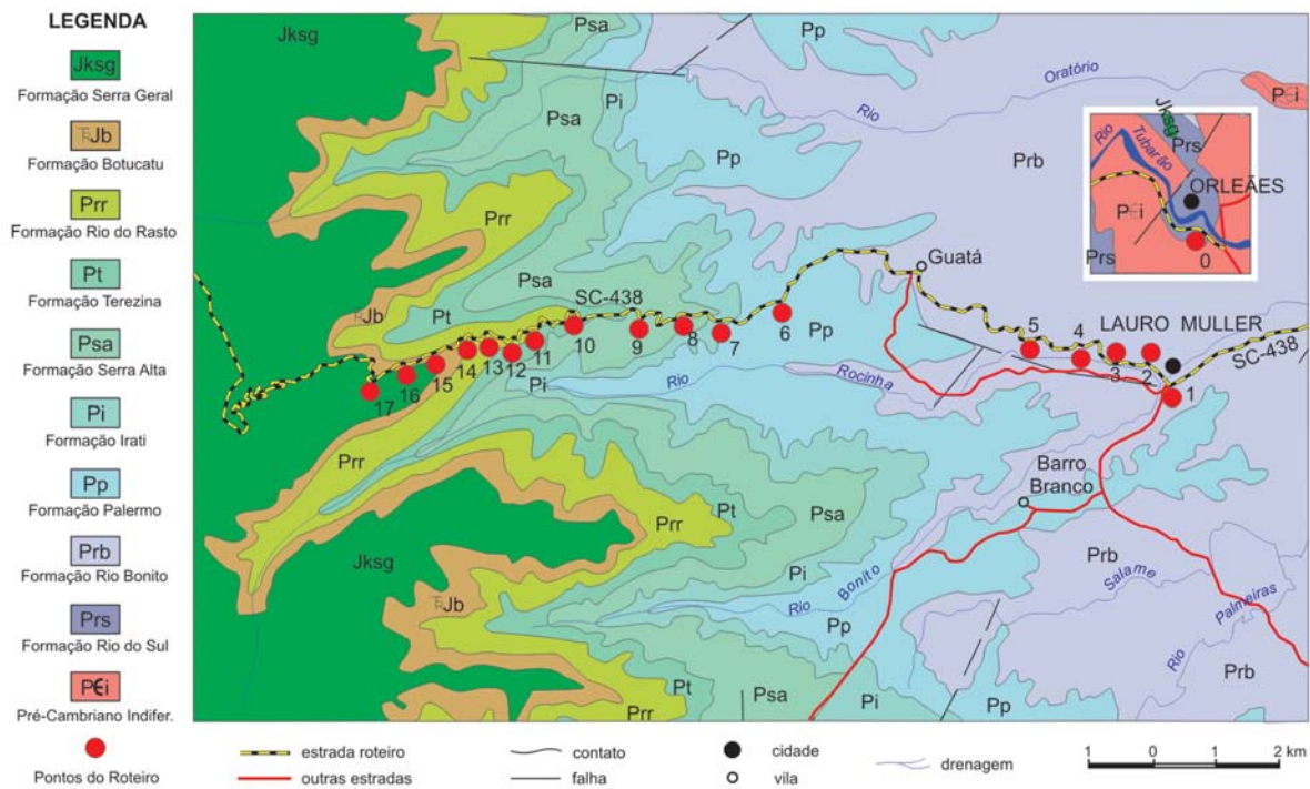
Figura 05 - Roteiro geológico da Serra do Rio do Rastro, com a indicação dos afloramentos demarcados.
