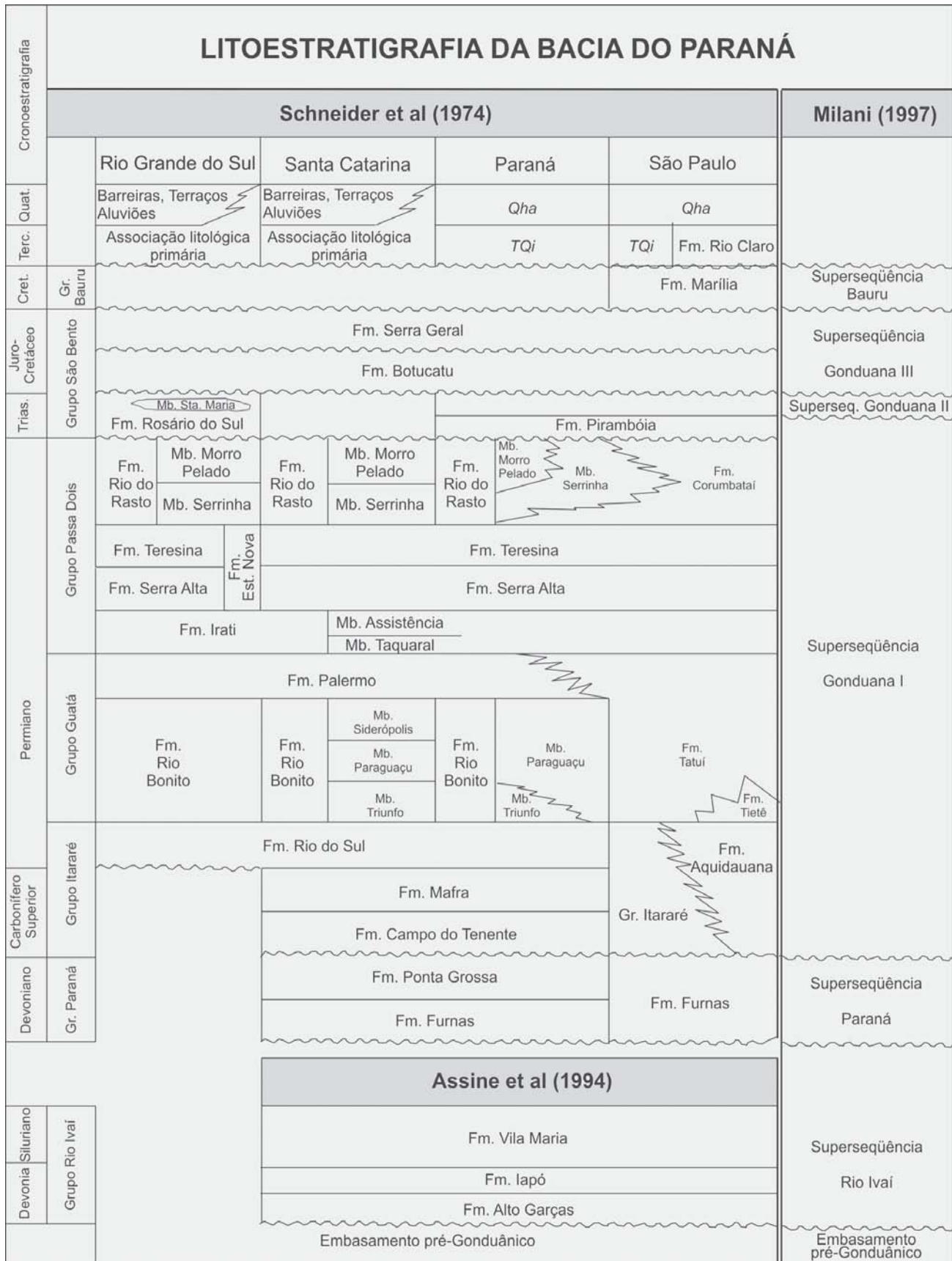
Figura 10 - Coluna estratigráfica da Bacia do Paraná, seg. Schneider et al. (1974) adaptada por Aboarrage e Lopes (1986), e correlacionada graficamente com atualizações de Milani (1997) e Assine (1994), conforme Lopes et al (2003).
