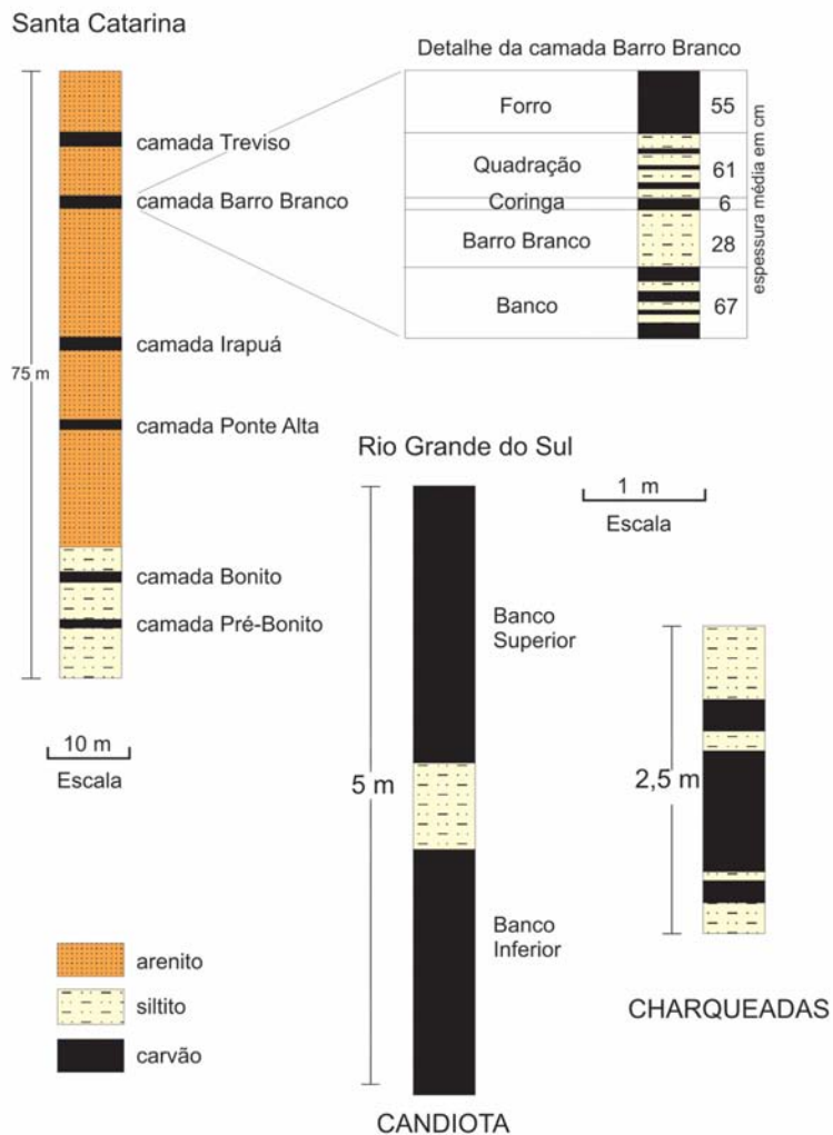
Figura 14 - Principais camadas de carvão no Rio Grande do Sul e Santa Catarina (adaptado de: Brasil. CPRM - Pesquisa de Carvão no Brasil,, 1972).
