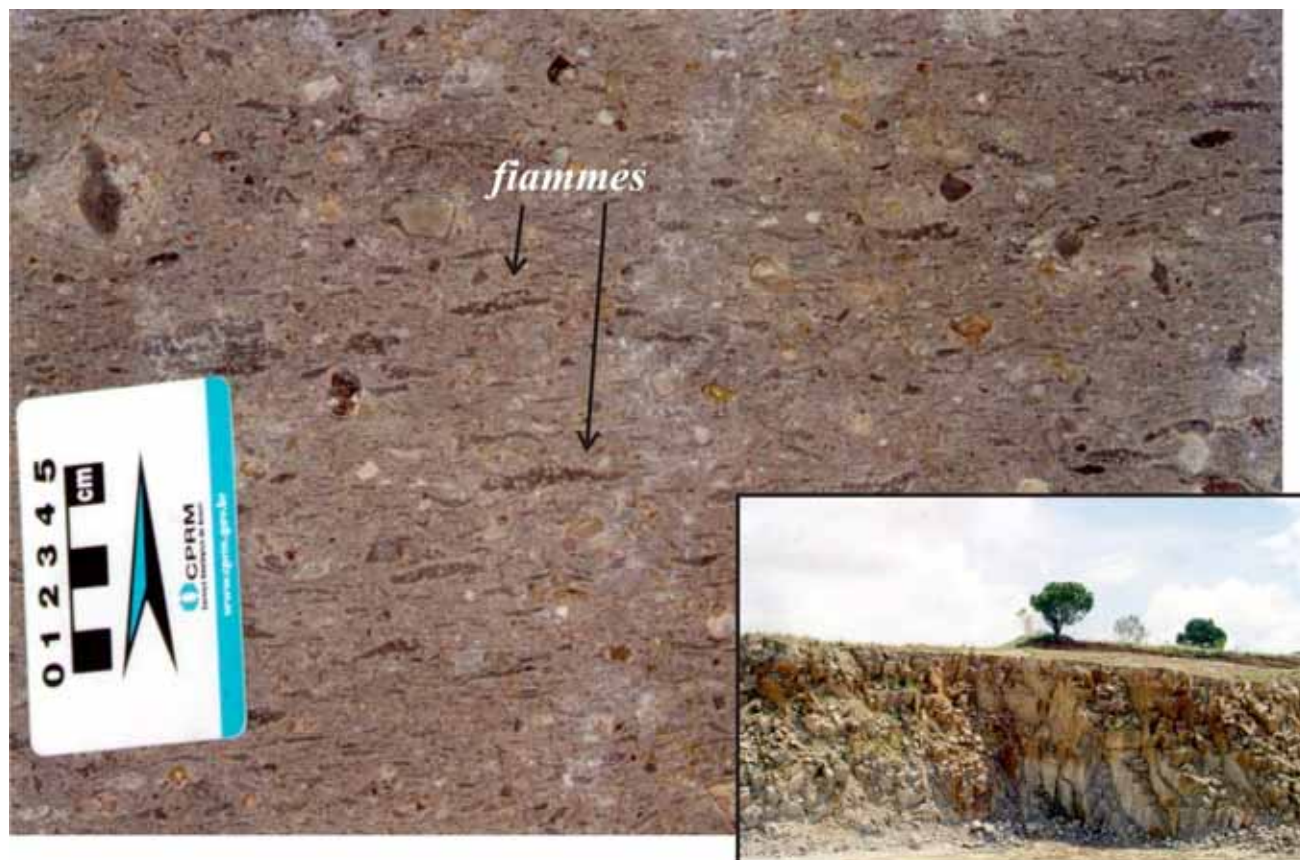
Figura 1 – Aspecto de campo do ignimbrito fortemente soldado com fragmentos juvenis ( fiammes ) gerando uma superfície plana. Figura 1A – Visão parcial da pedreira do Engenho Saco.
