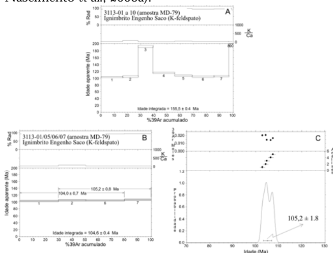
Figura 8 – Idades ^{40}\text{Ar} - ^{39}\text{Ar} (desvios de 2\sigma ) obtidas em feldspatos nos ignimbritos.
