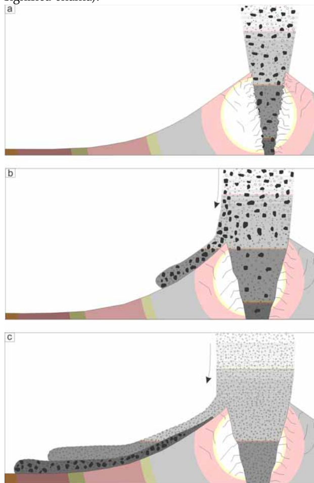
Figura 9 – Desenho esquemático mostrando os processos de geração de brechas líticas e ignimbritos. Modificado de Arnosio (2002). (a) Durante a evolução do ciclo magmático será produzida uma erupção altamente explosiva. Esta provocará a erosão do conduto e da boca de emissão, gerando elevada proporção de fragmentos líticos. (b) A erosão do conduto e a elevada quantidade de líticos conduz o colapso da coluna eruptiva e formação do fluxo piroclástico enriquecidos em líticos (brechas líticas). (c) A erupção continua emitindo material de grãos mais finos, formando ignimbritos que se depositam sobre as brechas líticas.
