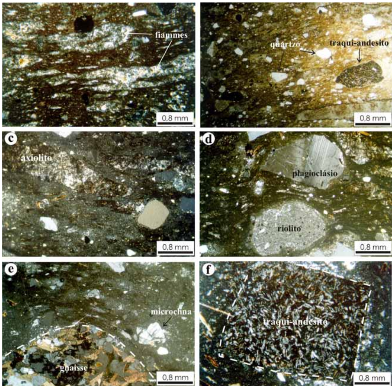
Figura 5 – Feições microscópicas dos ignimbritos. (a, b) Superfície planar (textura eutaxítica) definida pelos fiammes e cristaloclastos (quartzo e opacos). (c) Axiolito (vesículas, parcialmente achatadas, preenchidas por minerais secundários – quartzo e carbonatos) como produto de devitrificação em alta temperatura. (d) Fragmentos de plagioclásio e riolito fino. (e) Fragmento de rocha do embasamento pré-cambriano (gnaisse). (f) Fragmento de traqui-andesito com textura pilotaxítica.
