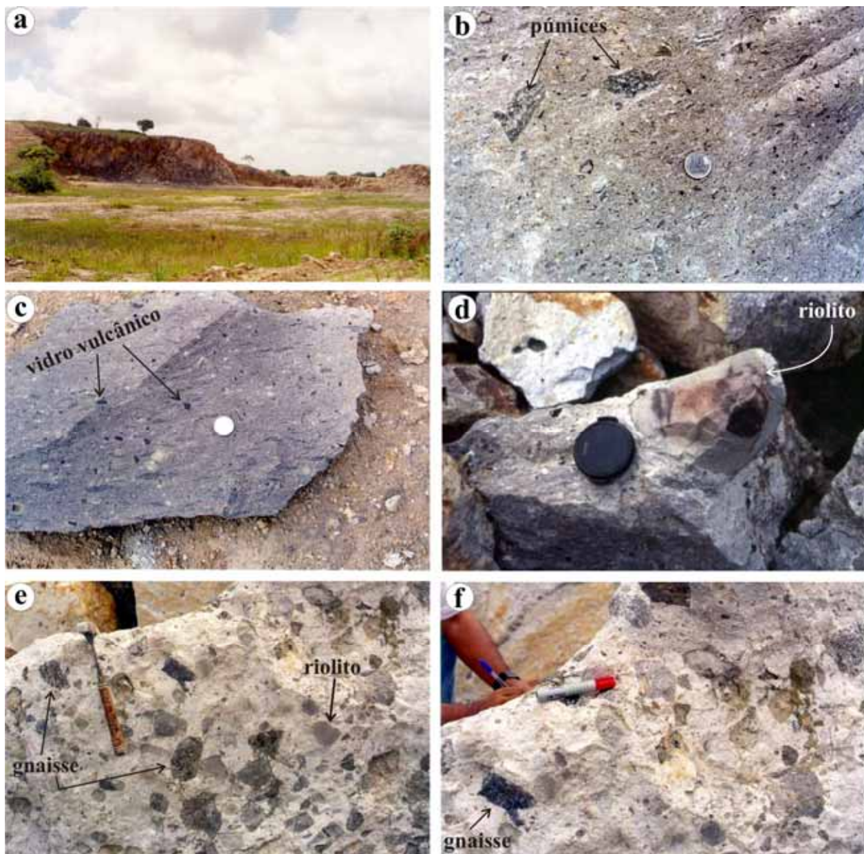
Figura 4 – Aspectos de campos das rochas ignimbríticas. (a) Visão geral da Pedreira do Engenho Saco com espessura média aflorante de 30 m de altura. (b, c) Ignimbritos fortemente soldados, com púmices (b) e vidro vulcânico (c) definindo superfícies planares. (d) Fragmento decimétrico de riolito de textura fina em ignimbritos da fração bomba. (e, f) Fragmentos milimétricos a decimétricos de rochas do embasamento pré-cambriano (gnaisse e granitos) e vulcânicas (riolitos e traquiandesitos).
