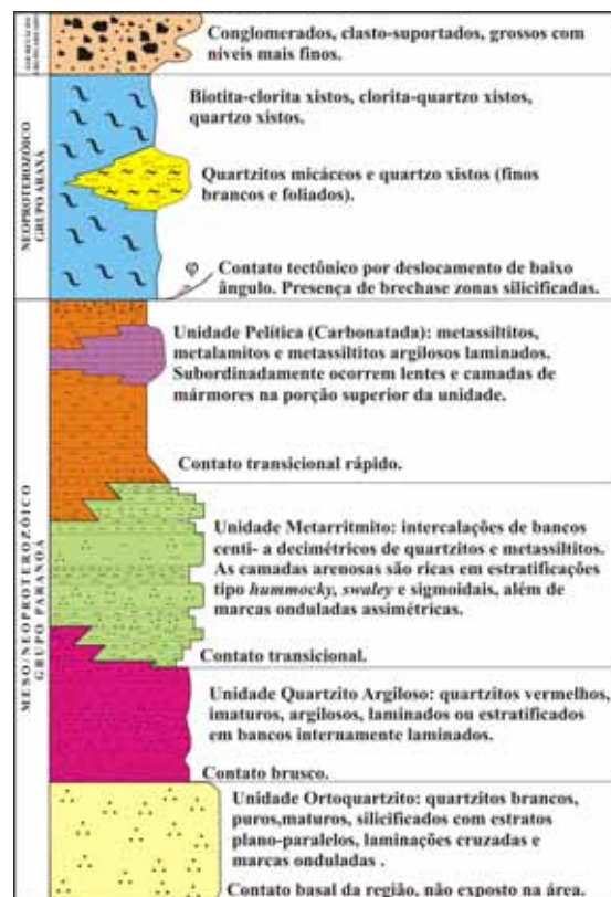
Figura 4 – Estratigrafia da região das águas termais do sudeste do estado de Goiás.
