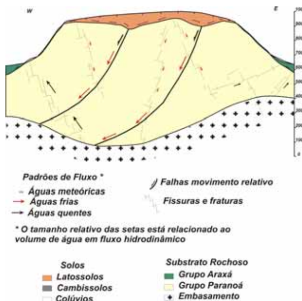
Figura 6 – Seção esquemática ilustrando os sistemas de fluxo hidrogeológico presentes na região das águas quentes do sudeste do estado de Goiás.
