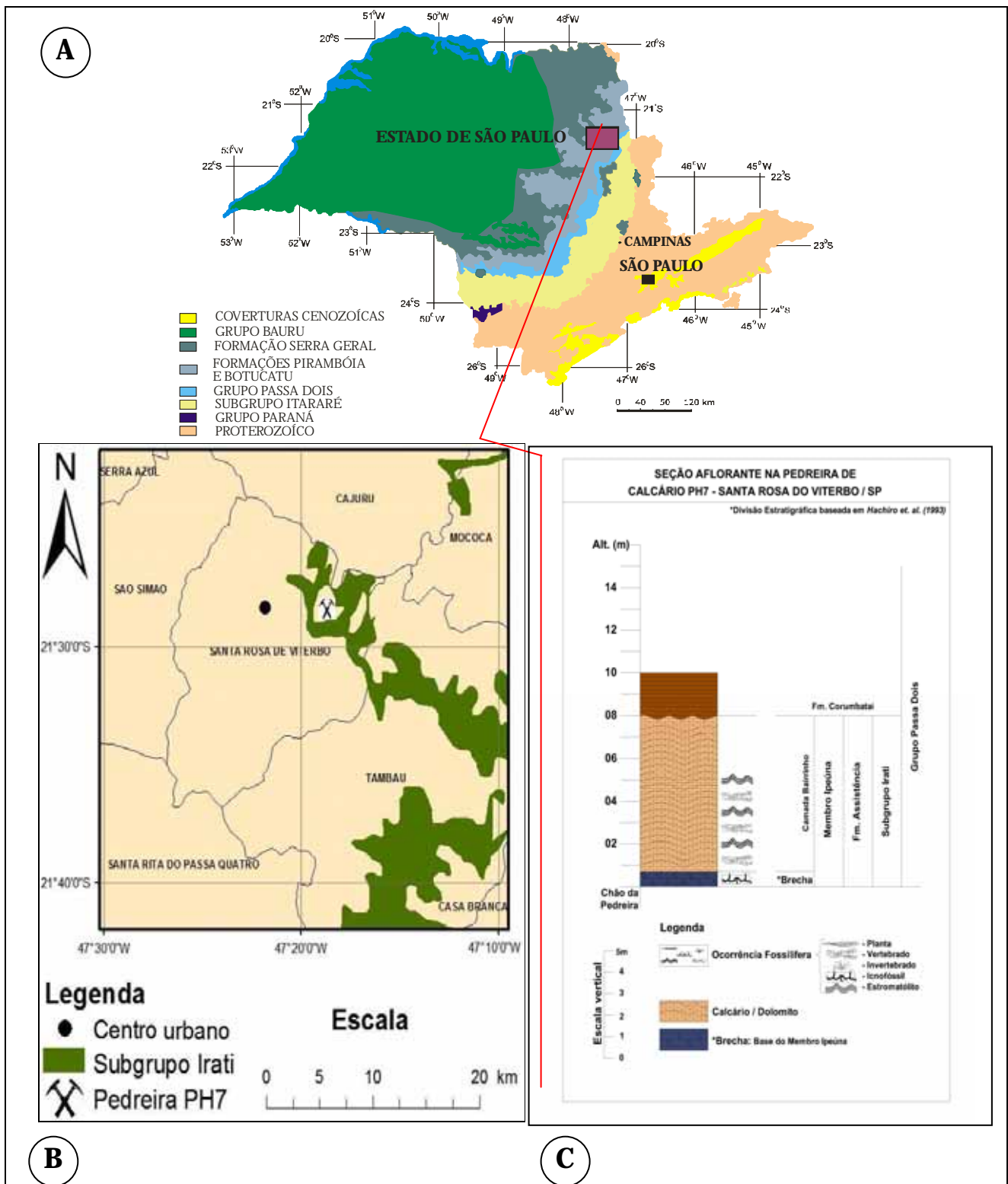
Figura 2 – Localização de Santa Rosa de Viterbo (A), da pedreira PH 7 (B) e coluna estratigráfica (C).
