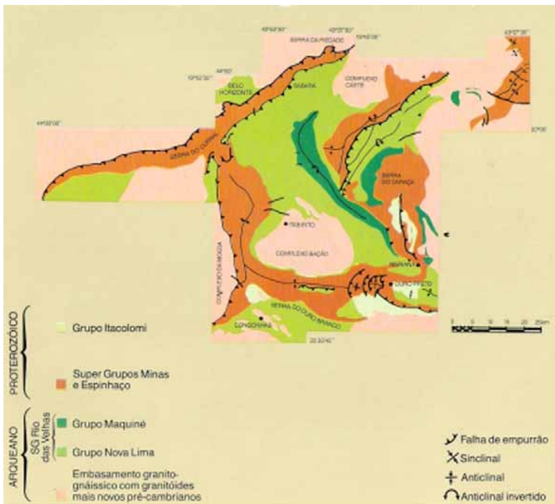
Figura 10 - Mapa geológico simplificado do Quadrilátero Ferrífero, segundo Dorr (1969). Fonte: Scliar, 1992. Figure 10 - Simplified geological map of the Quadrilátero Ferrífero, modified after Dorr (1969). Source: Scliar, 1992
