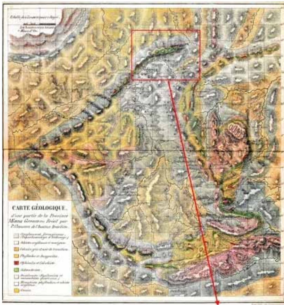
Figura 8 - Mapa geológico do Quadrilátero Ferrífero de P. Claussen (1841), no detalhe a Serra da Piedade junto às cidades de Sabará e Caeté; em verde o chamado “siderocristo” (formação ferrífera).
